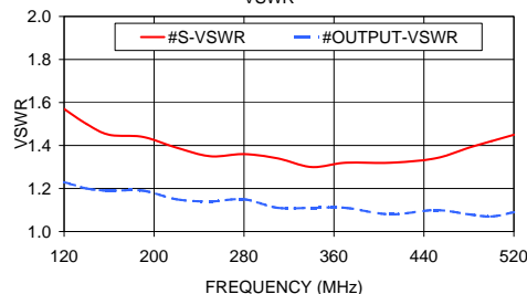
ZBSC-5-1 VSWR
