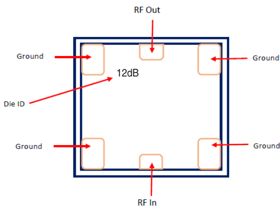
Fig 2. Die Layout
