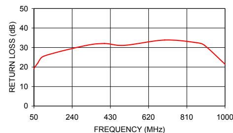
JTX-2-10TA+ INPUT RETURN LOSS
